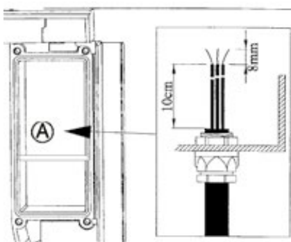
Boîtier de raccordement électrique
